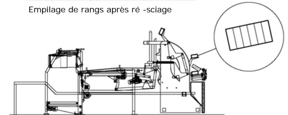
Empilage à grande capacité, jusqu'à 500 planches/min.
