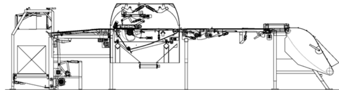
L'installation d'empilage comprend une tronçonneuse multi-lames de rangs, pour une capacité plus élevée
