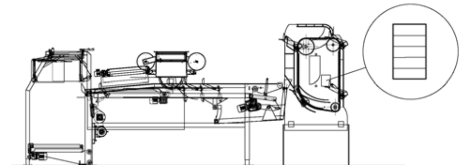
Cerclage de paquets de planches séparément avant empilage
