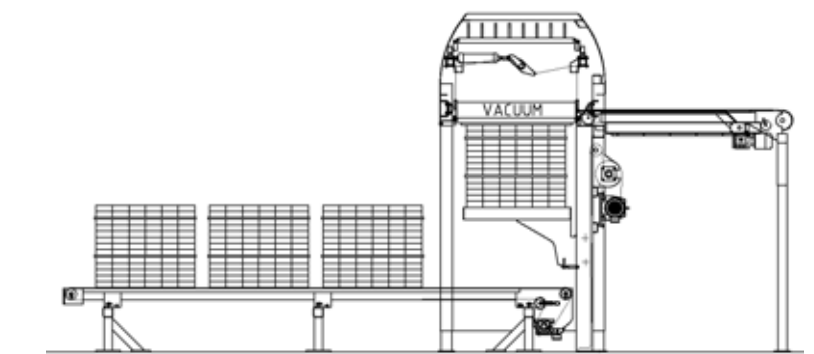
Dépilage en rangs transversalement, à vide par contacteur de dépression
